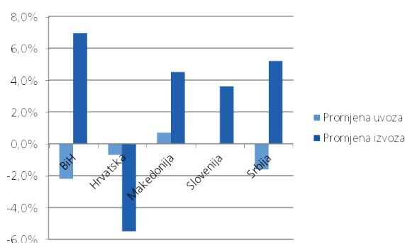
Grafikon 1: TREND PROMJENE UVOZA I IZVOZA U NEKIM ZEMLJAMA REGIJE
